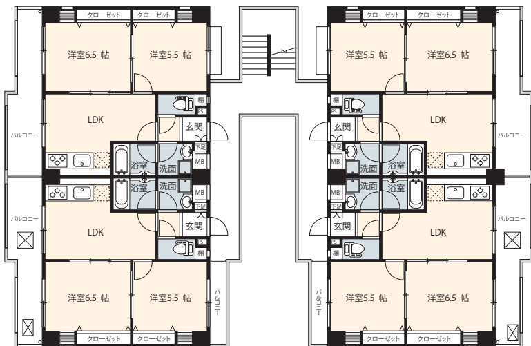
2階(201号室~204号室)・3階(301号室~304号室)平面図
